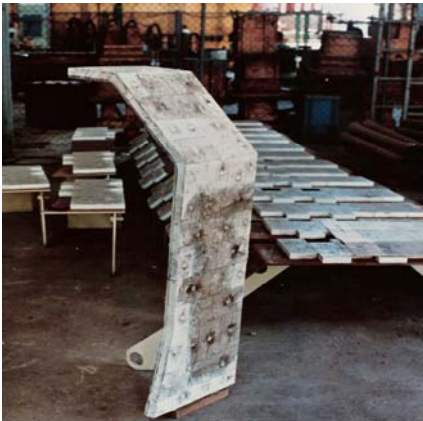
Riparo interno mulino
